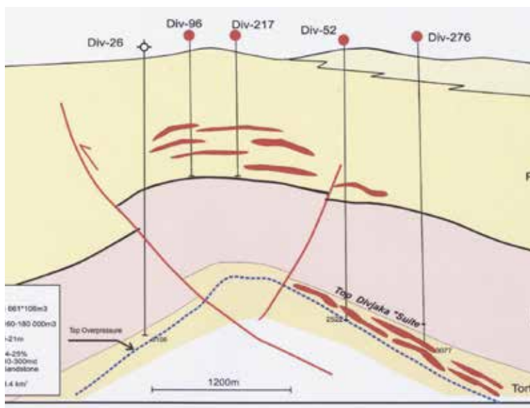
Fig. 12 Divjaka gasfield (sandstones)
